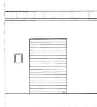
PROSPETTO OVEST
